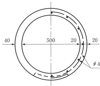
雨水側塊 500×500
