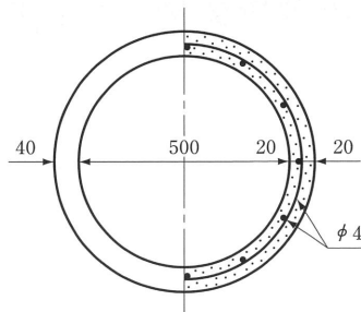
汚水側塊 500×400
