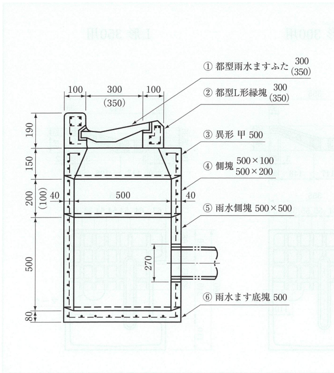
都型雨水ます (単位 m/m)
