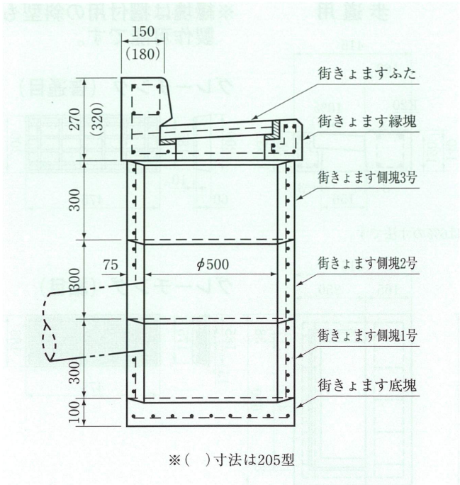
街きよ用集水ます (単位 m/m)
