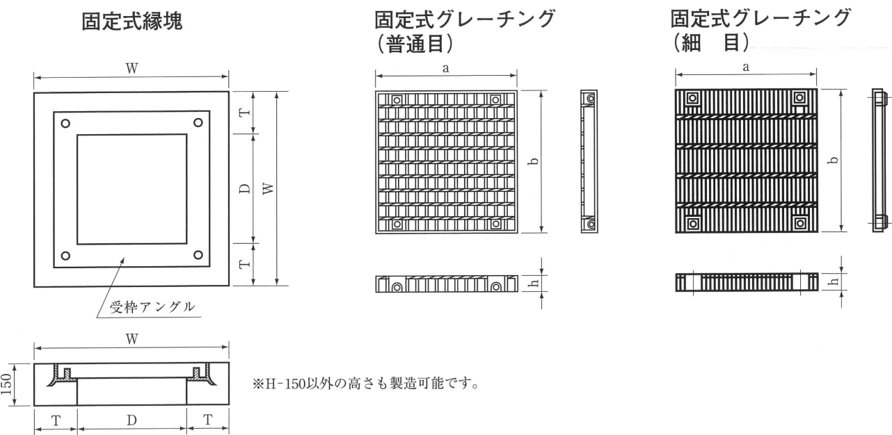
角型集水ます縁塊（ボルト固定枠付）
