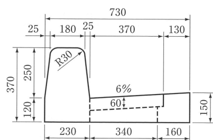
両面歩車道 C用
