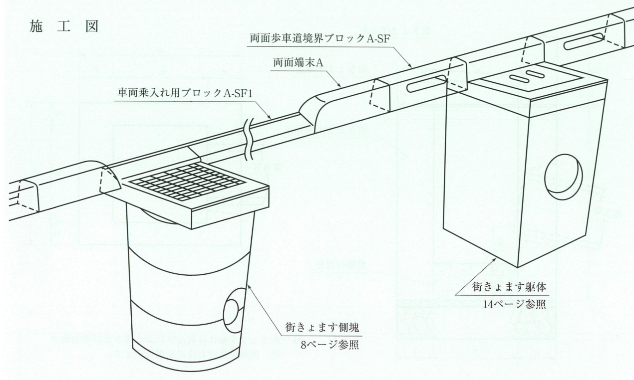
街きよます縁塊 車乗入れ
