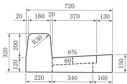
両面歩車道 B用
