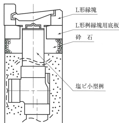
施工例
