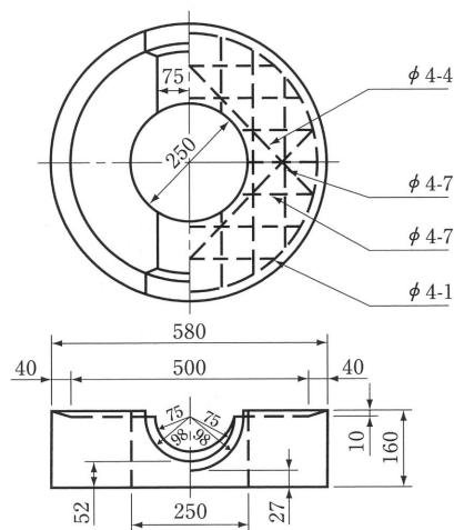
500用底部有孔
