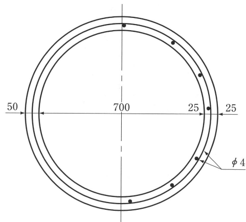
内径 70cm
