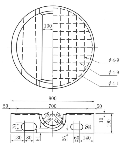
700用
