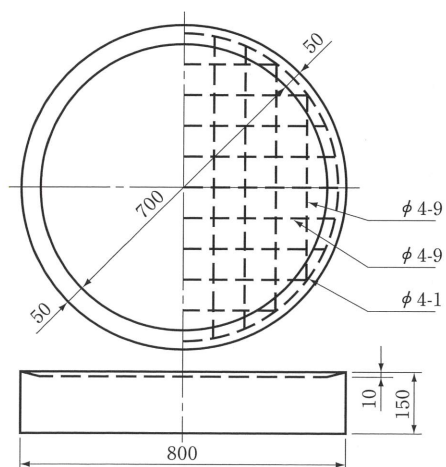
700用(フラット)
