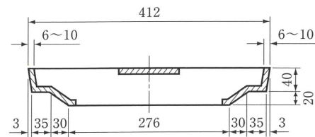
X~X断面
