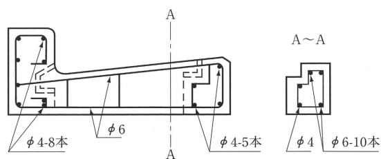
配筋図
