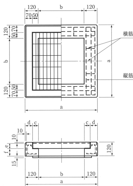
グレーチング用 (落し込みタイプ・ボルト固定式タイプ)
