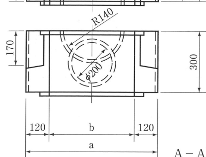
A-A' 断面
