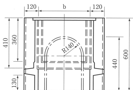
上部側塊
