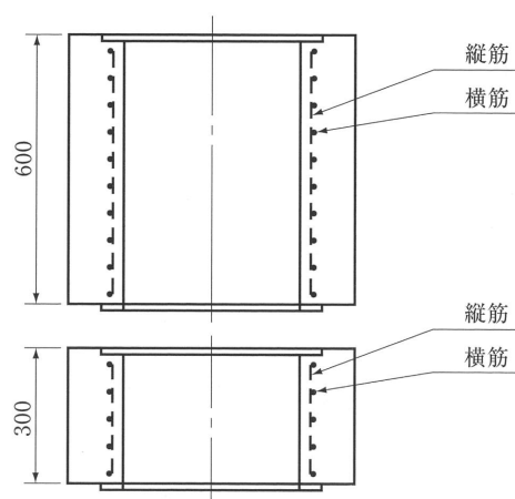
B-B' 断面
