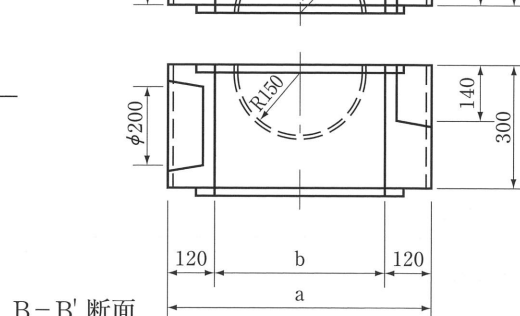
B-B' 断面
