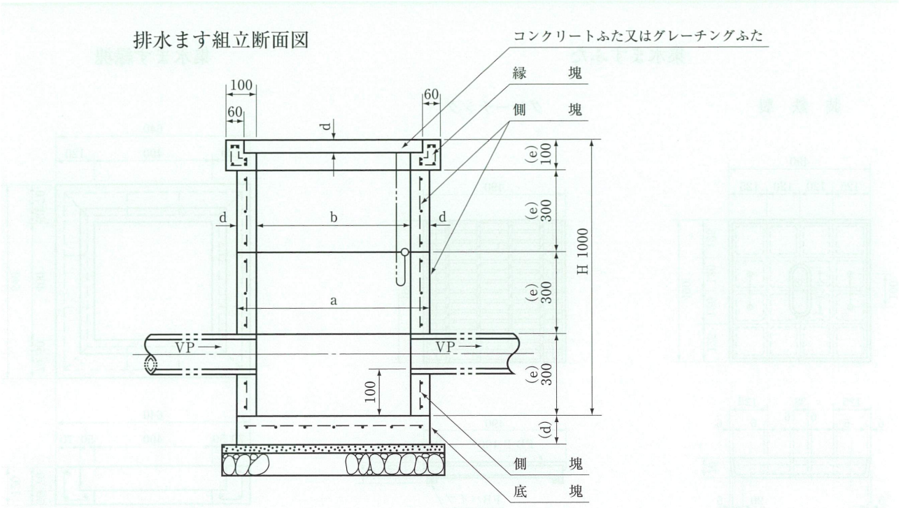
鉄筋コンクリート汚水ます・排水ます（CD型） (単位 m/m)
