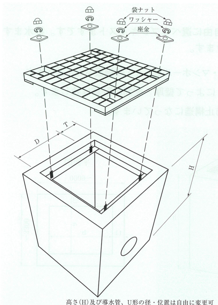
角型集水ます
