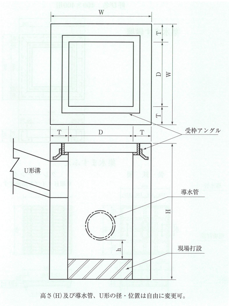
角型集水ます
