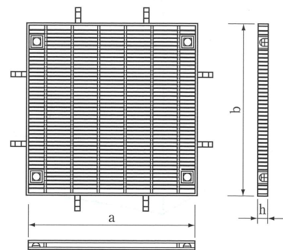
(細目) 表面ノンスリップ加工品
