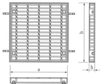
(細目) 表面ノンスリップ加工品
