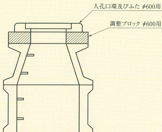
組立て構造図
