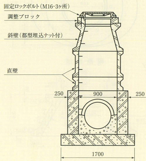
楕円形人孔（内径120cm×90cm）
