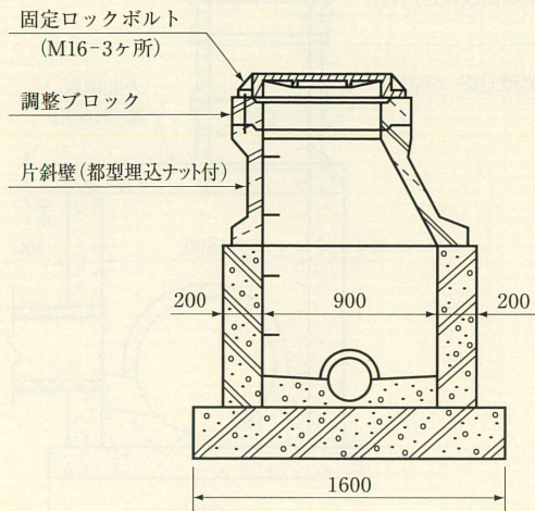
円形人孔（内径90cm）
