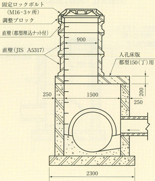
円形人孔（内径150cm丁）
