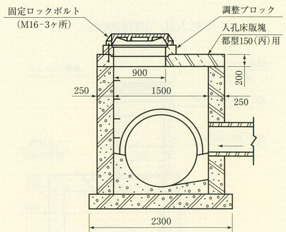
円形人孔（内径150cm丙）
