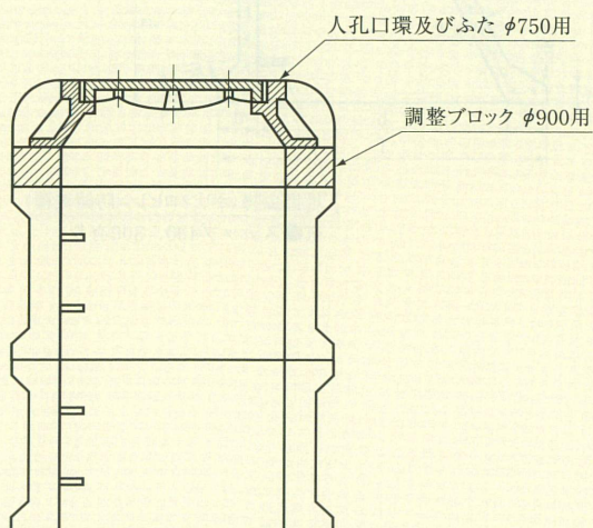
組立て構造図
