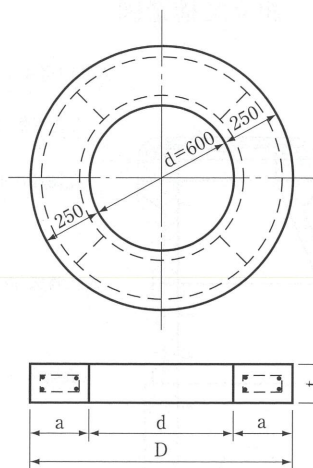
調整ブロック \phi 600 用
