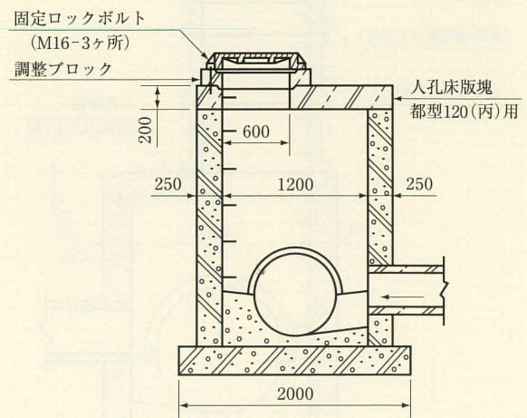
円形人孔（内径120cm丙）
