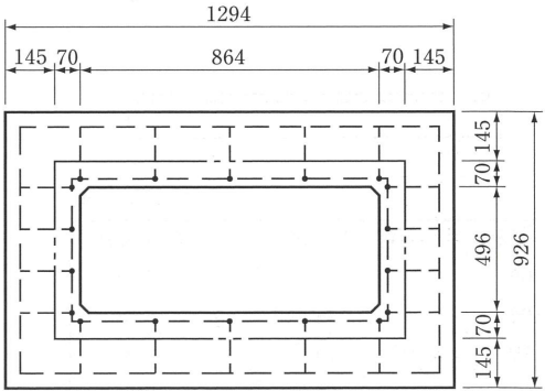
双口消火栓ブロック (単位 m/m)
