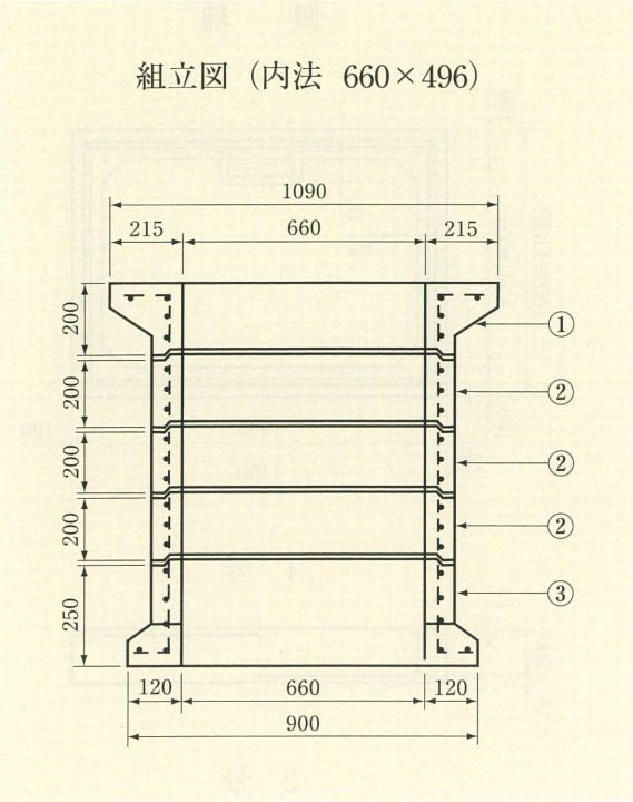
単口消火栓ブロック (単位 m/m)
