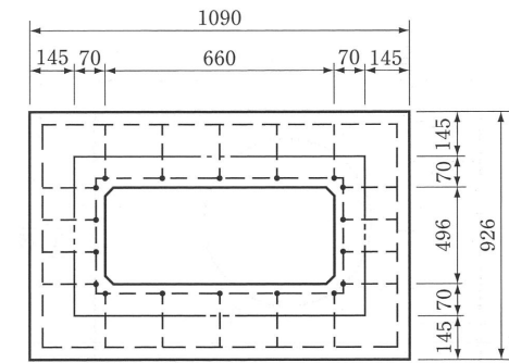
単口消火栓ブロック (単位 m/m)
