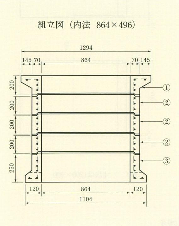
双口消火栓ブロック (単位 m/m)
