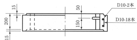
直壁 高 20cm
