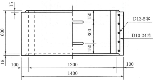
直壁 高 60cm
