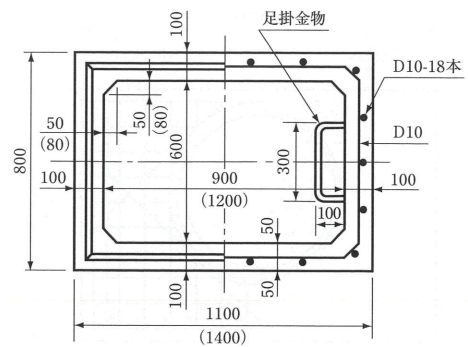
直壁 高 20cm
