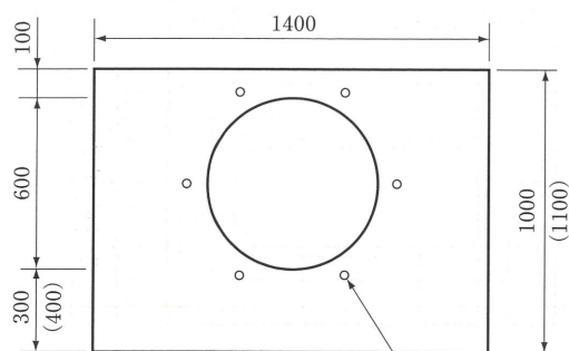
床 版
