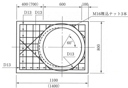
床版
