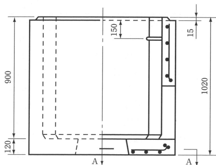
管取り付壁
