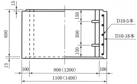
直壁 高 60cm
