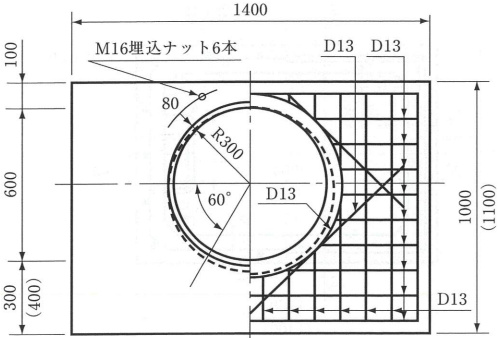
床版
