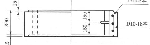
直壁 高 30cm
