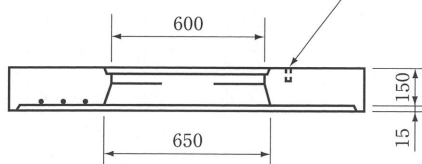
底 版
