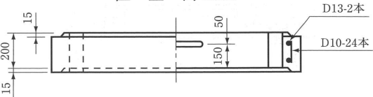
直壁 高 30cm
