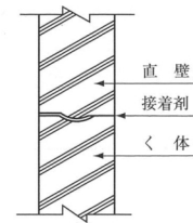
直壁・躯体ブロックの接合部
