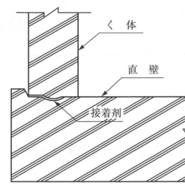
躯体ブロック・底版の接合部
