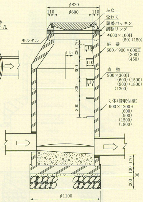
縦断面図
