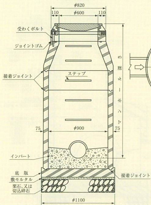
横断面図
