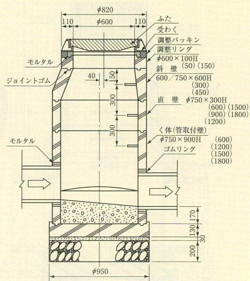
縦断面図
