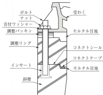
受わく・調整リング・斜壁の接合部
