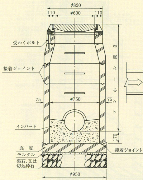
横断面図
