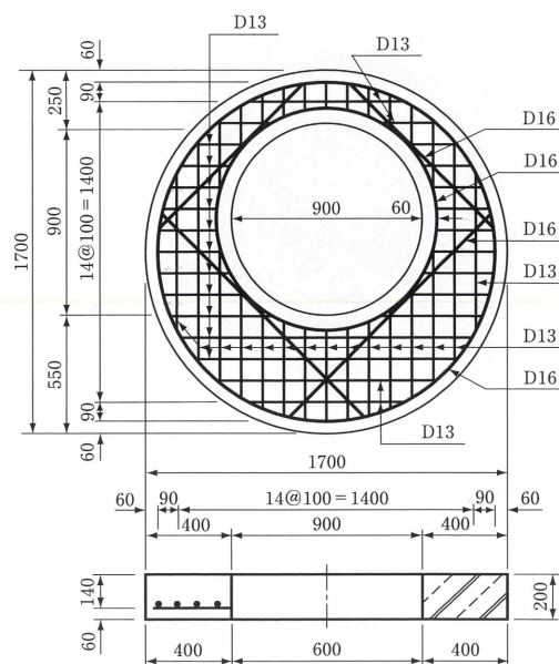
都型円形用人孔床版（内径 120cm 丁）
