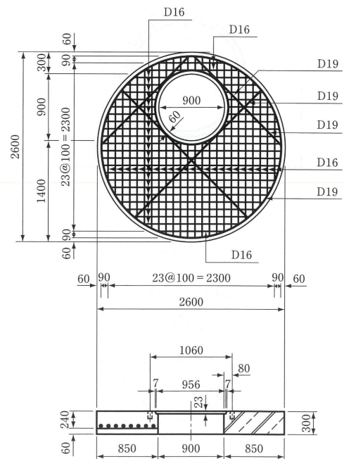
都型円形用人孔床版 (内径 200cm用) (埋込ナット付)
