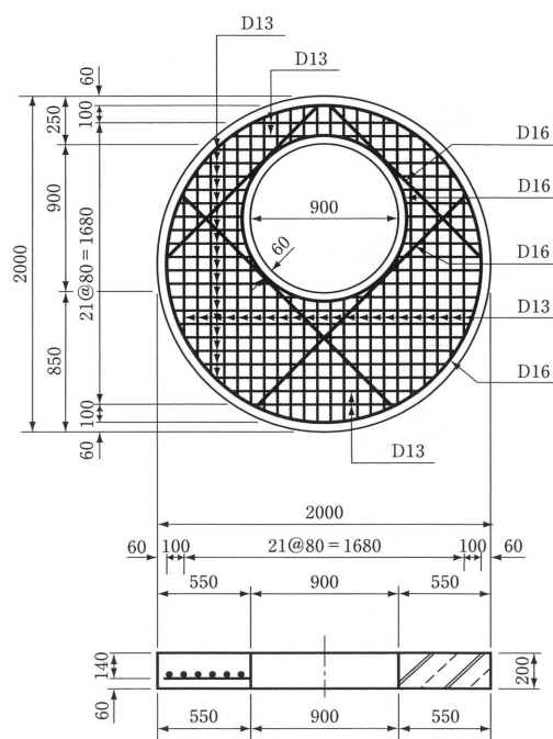
都型円形用人孔床版（内径 150cm 丁）
