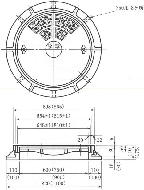
鑄鉄製人孔口環及びふた（単位 m/m）
