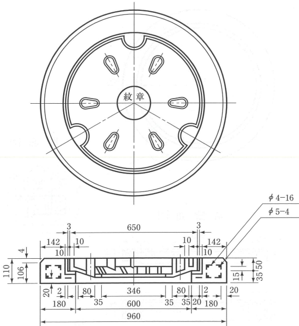
装鉄製人孔口環及びふた（単位 m/m）
