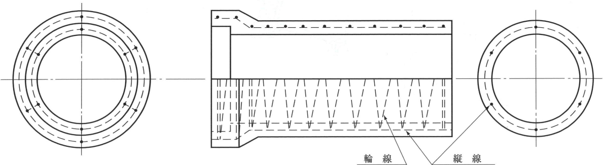
鉄筋配筋図
