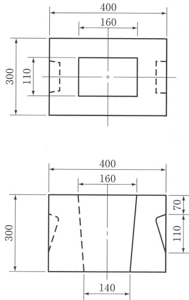
ガードレール ブロック (単位 m/m)
