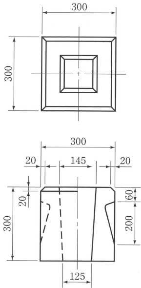
ガードレール ブロック (単位 m/m)
