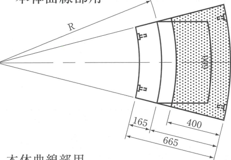
プレキャスト街きょ 本体曲線部用
