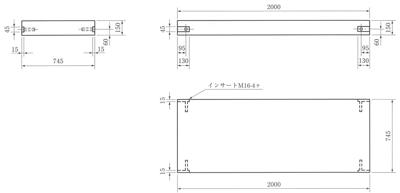
受 台
