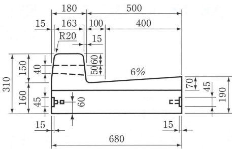
一般部水抜き 1ヶ所 (曲線部用も有り)
