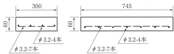
受 台
