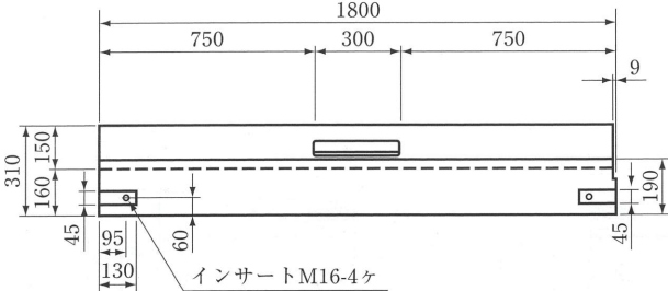
一般部水抜き 1ヶ所 (曲線部用も有り)
