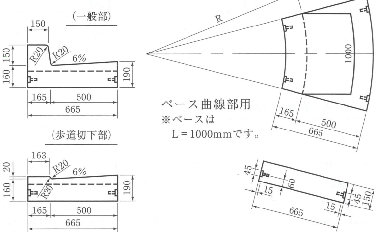
プレキャスト街きょ ベース曲線部用
