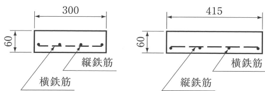
受 台
