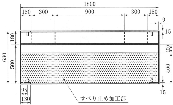
一般部水抜き 2ヶ所 (曲線部用も有り)
