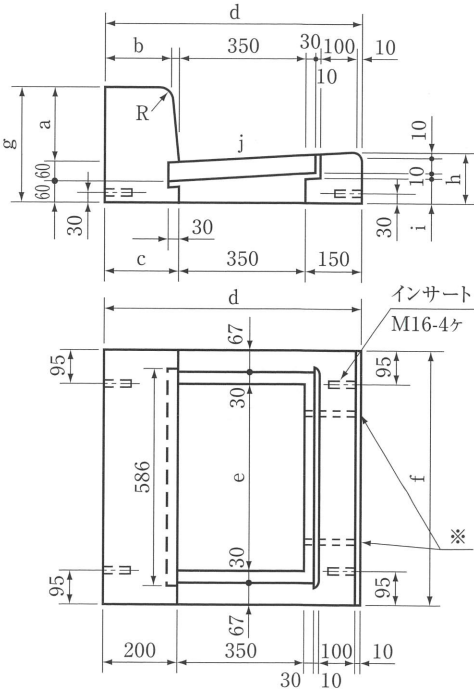
プレキャスト街きょ連結用 縁塊
