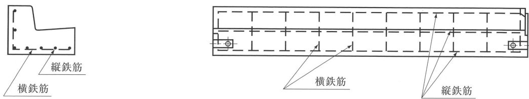
配 筋 図
