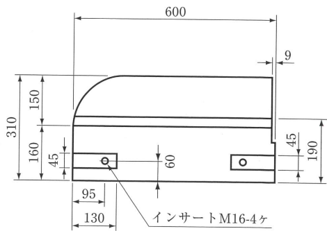
端末（右）
