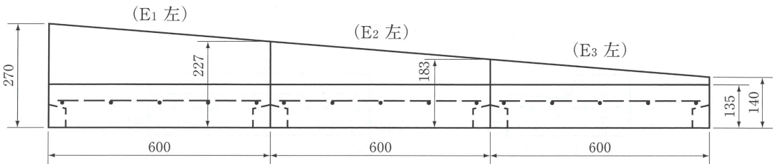
歩行者横断用 3 本下り E1、E2、E3 (右・左)
