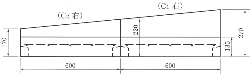
車乗入れ用 2 本下り C1、C2 (右・左)
