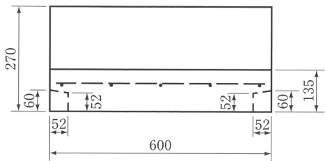
街築用特殊L形（A型）（105型）
