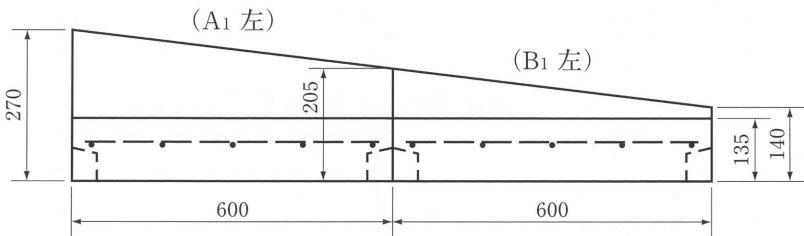
歩行者横断用 2 本下り A1、B1 (右・左)
