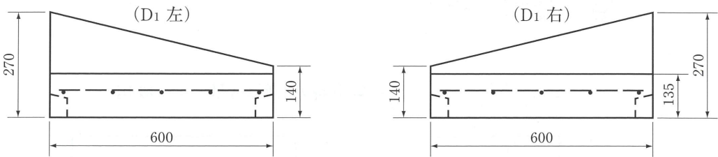
歩行者横断用 1 本下り D1 (右・左)
