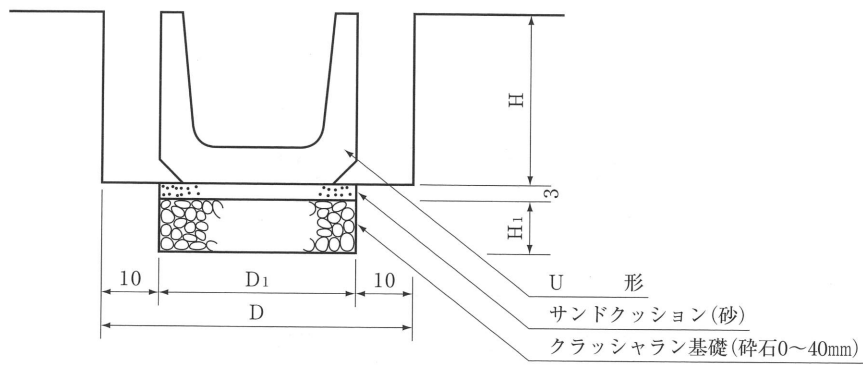
U形の敷設標準構造図（ふた掛けしない場合もしくは輪荷重量を受けないふた掛けの場合）
