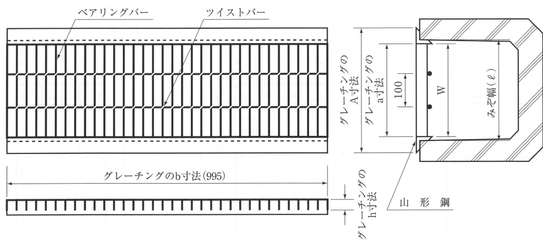
U形用グレーチングふた (単位 m/m)
