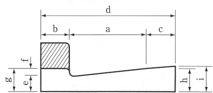
歩行者横断平坦部
