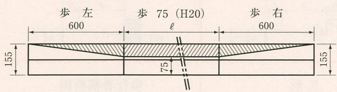
歩行者横断部左右（タイプ1）
