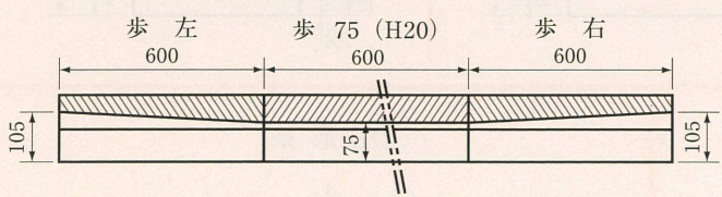
歩行者横断部左右（タイプ2）
