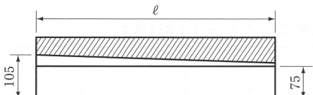
歩行者横断部切下げ（タイプ2）
