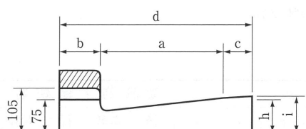
鉄筋コンクリートL形（歩行者横断用） (単位 m/m)
