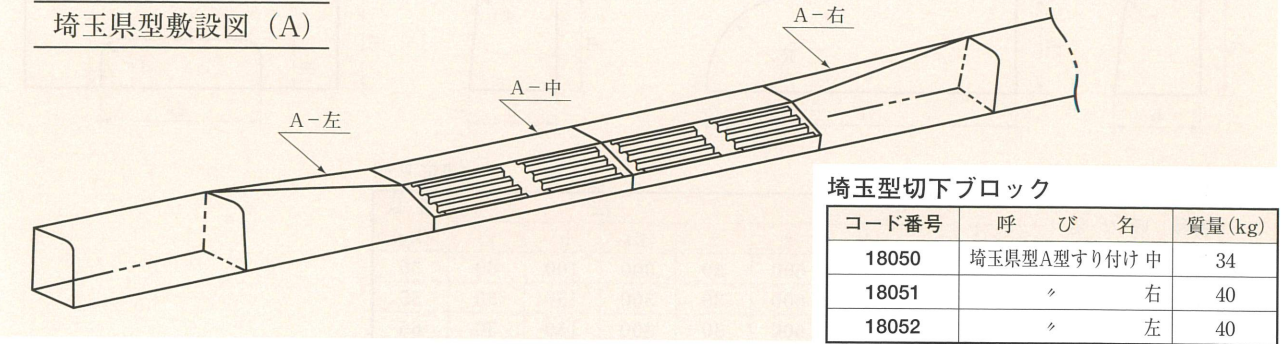
埼玉県型A-中
