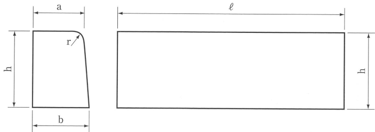
コンクリート特殊境界ブロック
