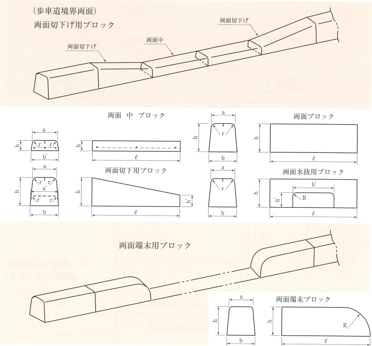
歩車道境界特殊コンクリートブロック
