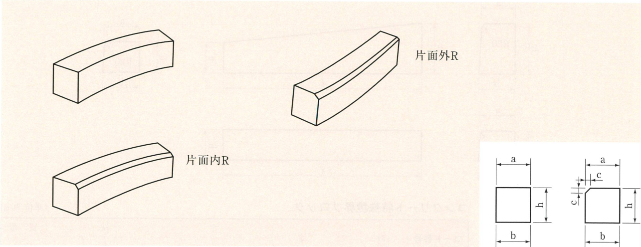
コンクリート境界ブロック曲線用 (単位 ㎡/m)
