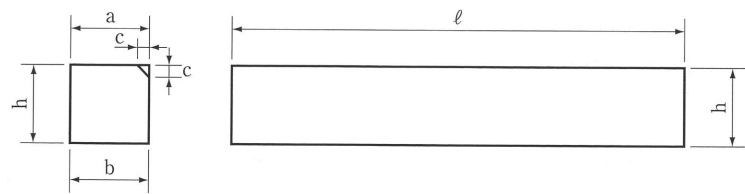
コンクリート特殊境界ブロック
