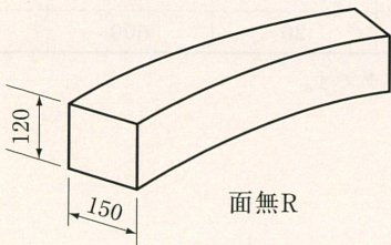
150×120×600 地先B
