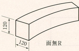
120×120×600 地先A
