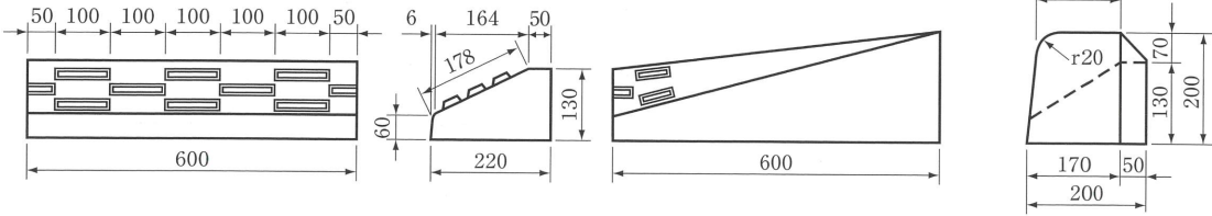
江戸川区型A-中
