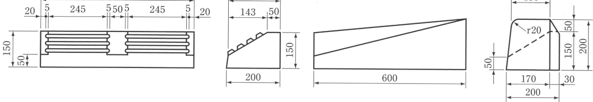
埼玉県型敷設図（B）
