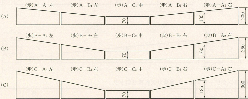
歩行者用横断ブロック (段差2本下り)
