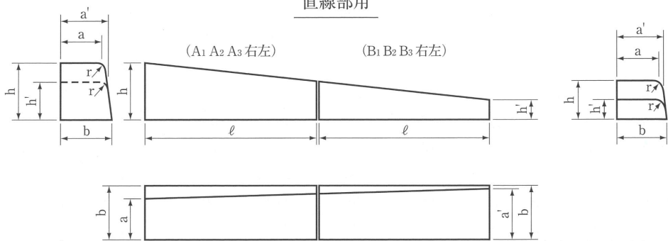
直線部用
