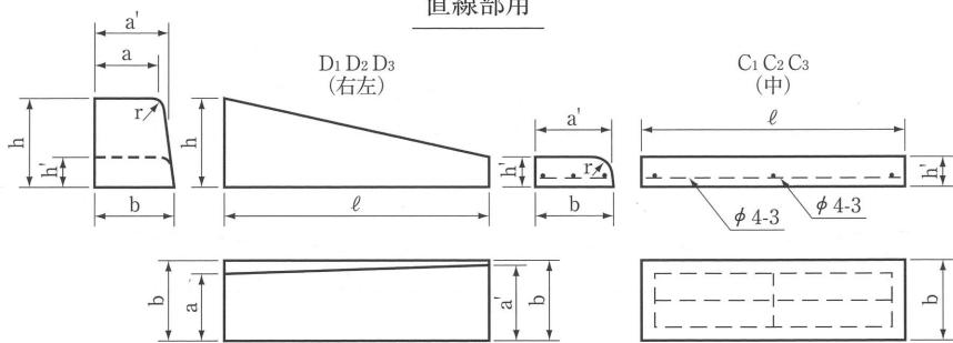
直線部用
