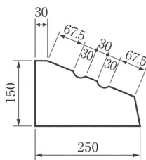
C-C' 断面
