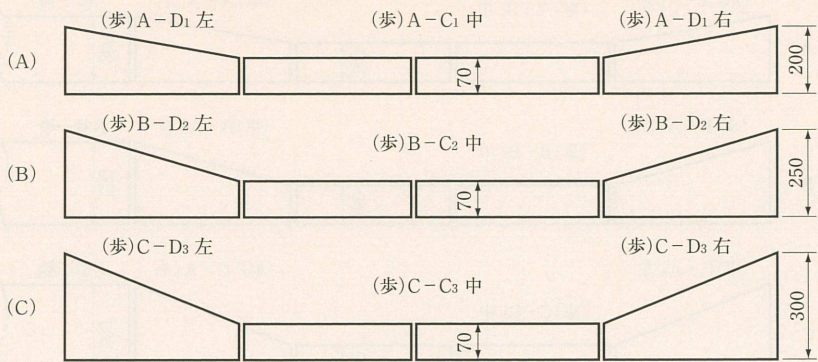
歩行者用横断ブロック (段差1本下り)
