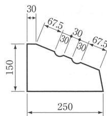
D-D' 断面
