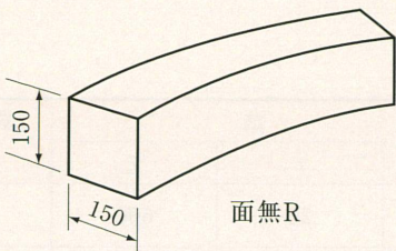
150×150×600 地先C
