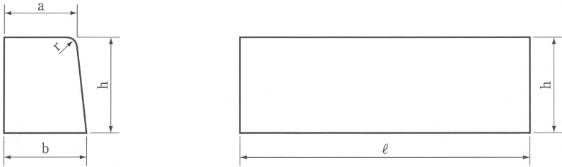
コンクリート歩車道境界ブロック
