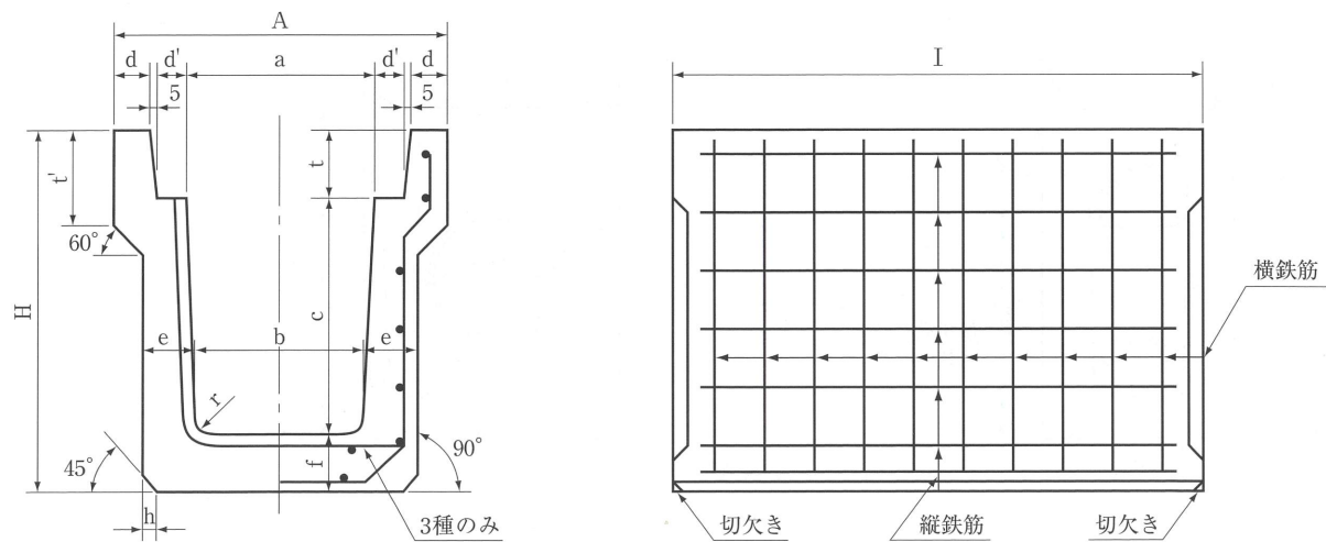
形状・寸法及び配筋 〈1種及び3種〉
