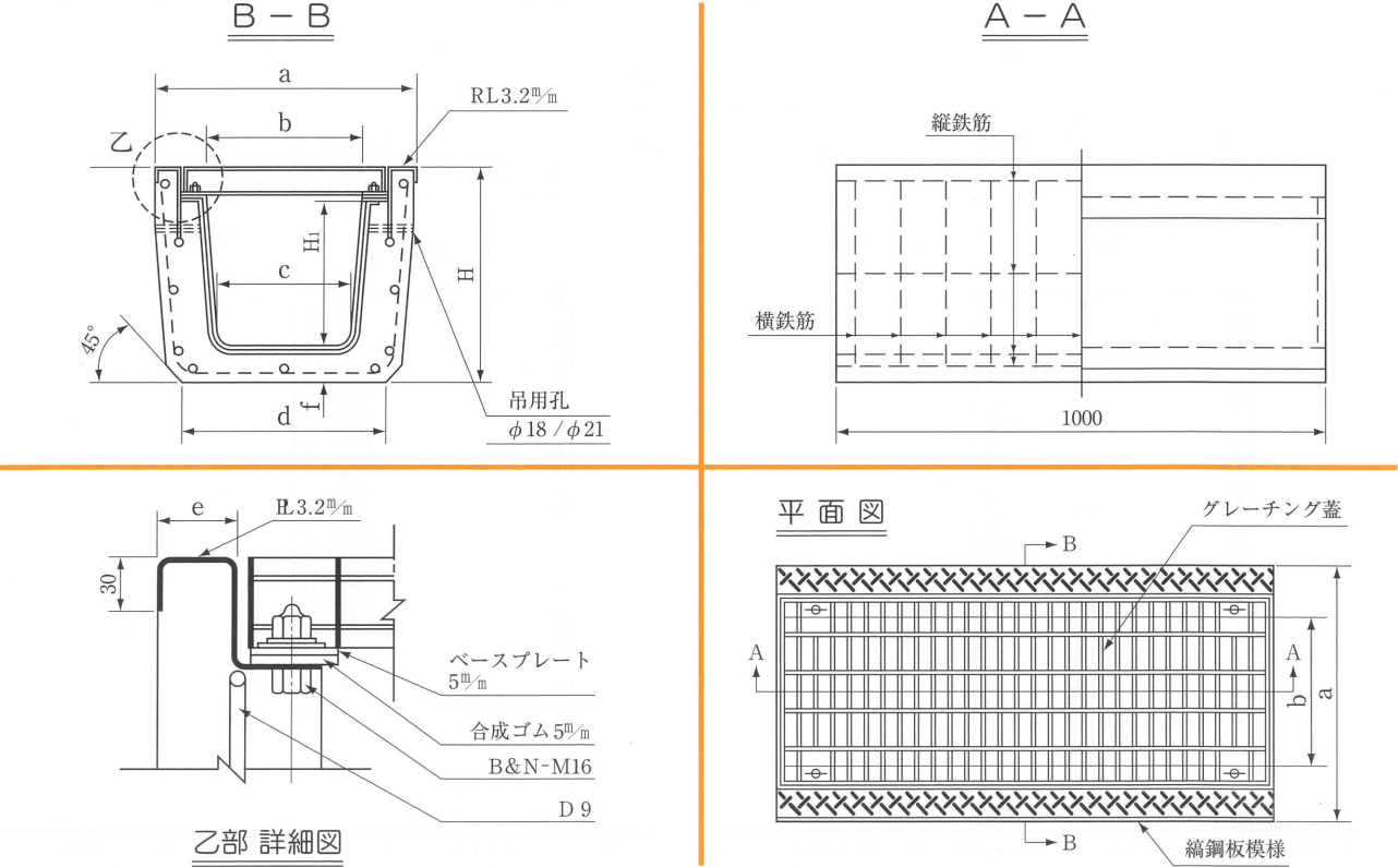
横断用U形 T-25（グレーチング固定式） (単位 mm)
